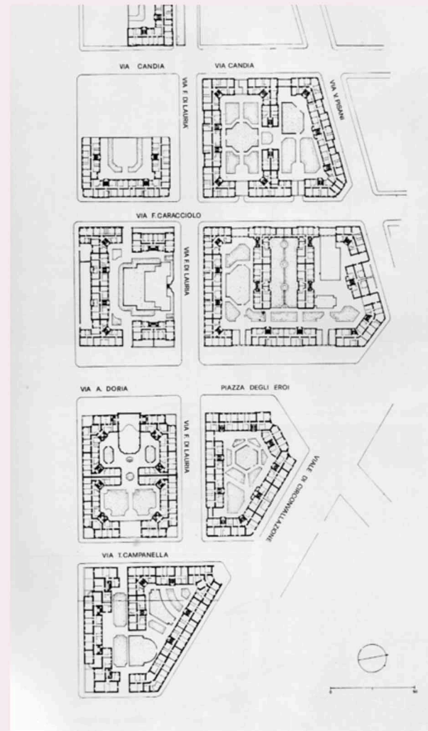
Planimetria ICP Trionfale.
